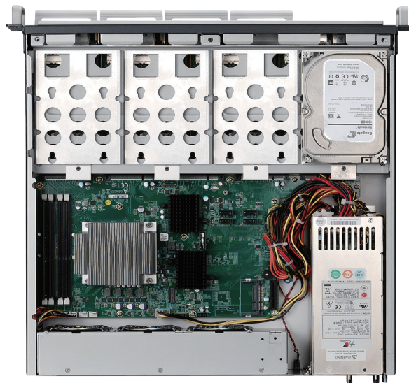
顶视图
